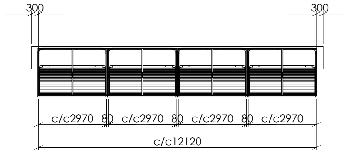
FRONTVY
