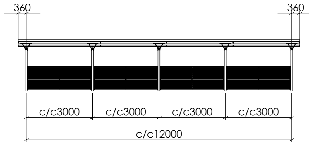
FRONTVY
