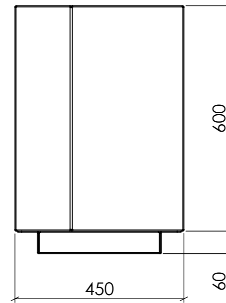
SIDOVY
