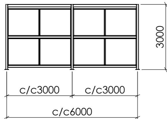
FRONTVY
