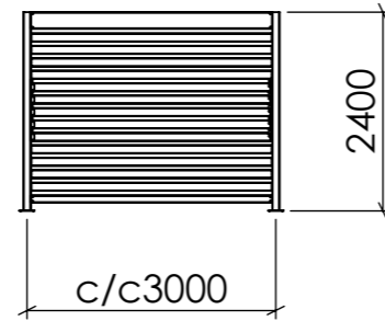
FRONTVY
