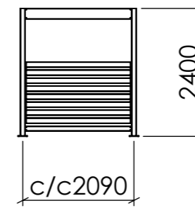
SIDOVY
