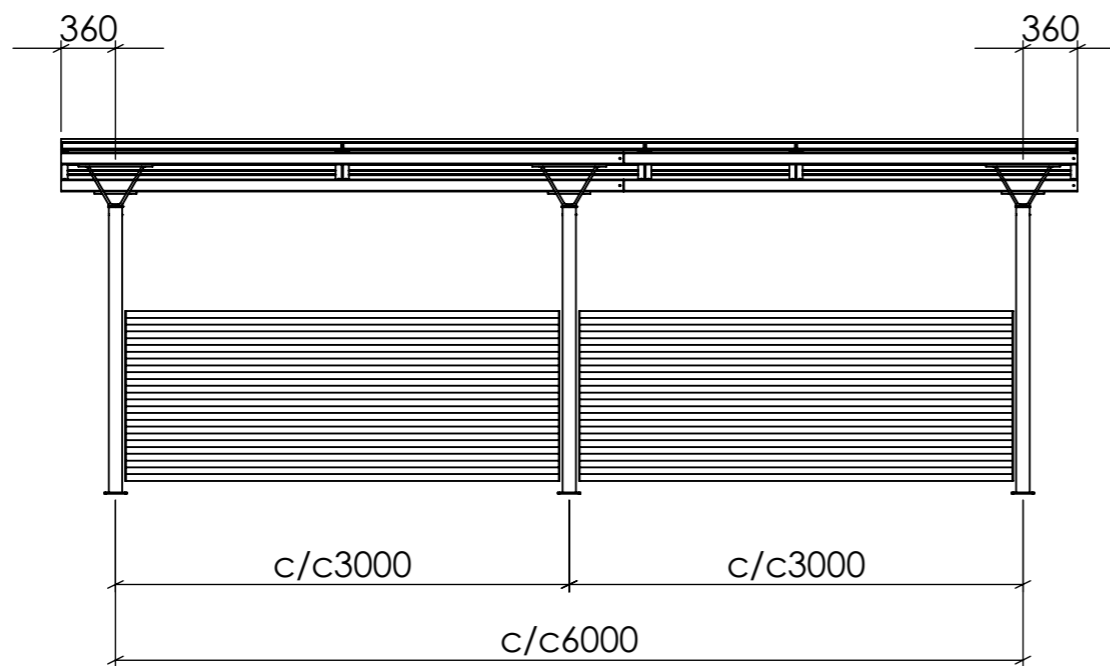
FRONTVY
