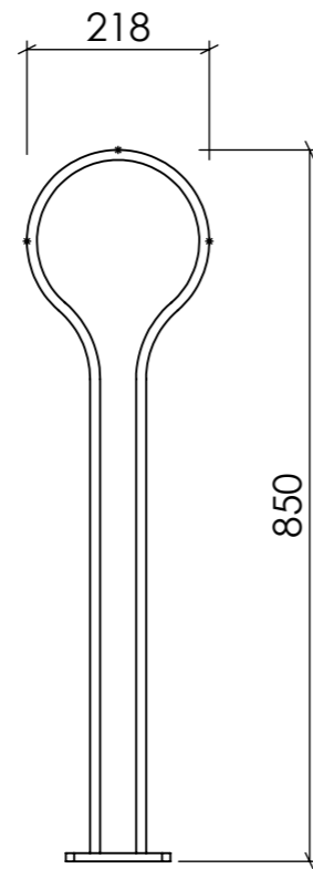
FRONTVY
